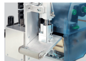
Anrollstempel
